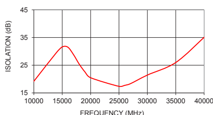
ZN2PD-K44+ ISOLATION
