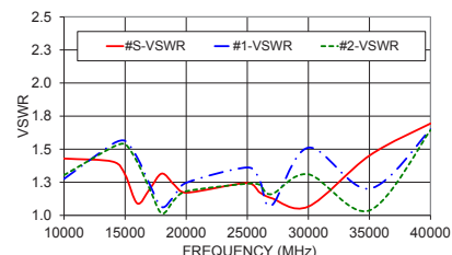
ZN2PD-K44+ VSWR
